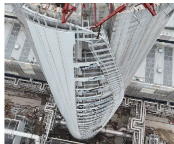
煙囪外牆飾板 安裝進行中
