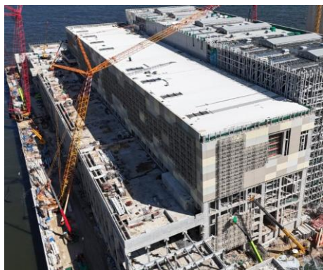
廢物儲存槽設備調試進行中，1號爐組試運行中
