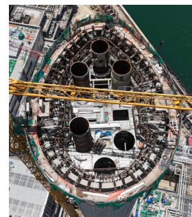
煙囪結構完成，鋼 平及台煙氣管道安 裝進行中
