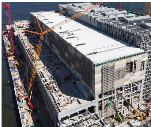
廢物儲存槽已完成，設 備安裝進行中
