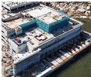
海水化淡廠結構 施工完成，設備 安裝調試進行中
