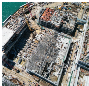
機械分類廠結構 施工進行中
